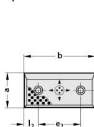
形式 D Shape D
