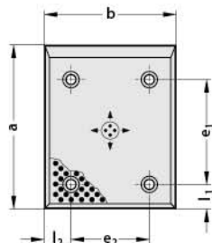
形式 D Shape D
